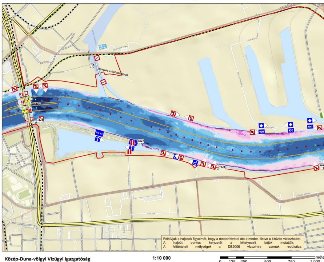
Hajóút kitűzési terv
