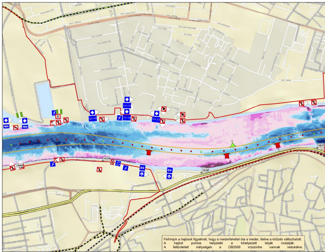
Hajóút kitűzési terv
